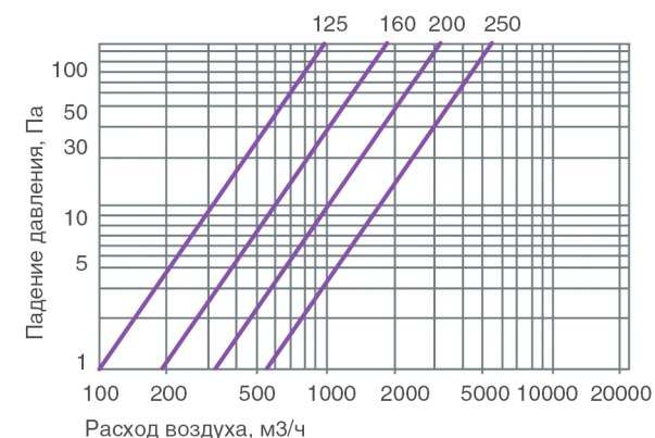
Круглые шумоглушители KS длиной 600 мм.
