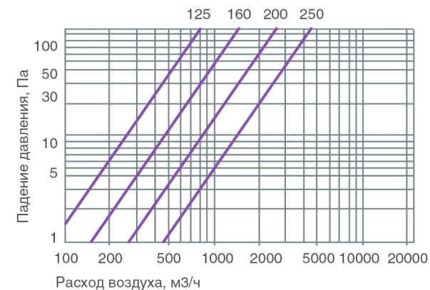
Круглые шумоглушители KS длиной 900 мм.
