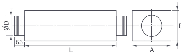
Круглые шумоглушители KS длиной 600 мм.
